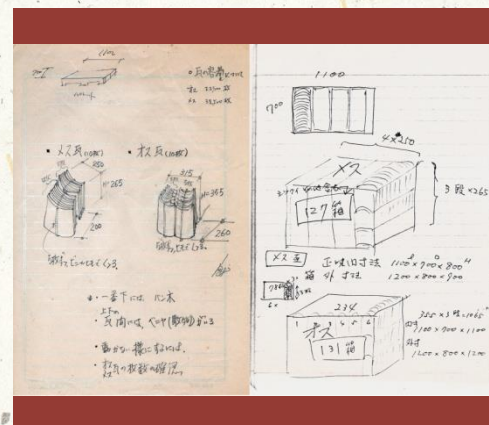
瓦の梱包イメージ図
